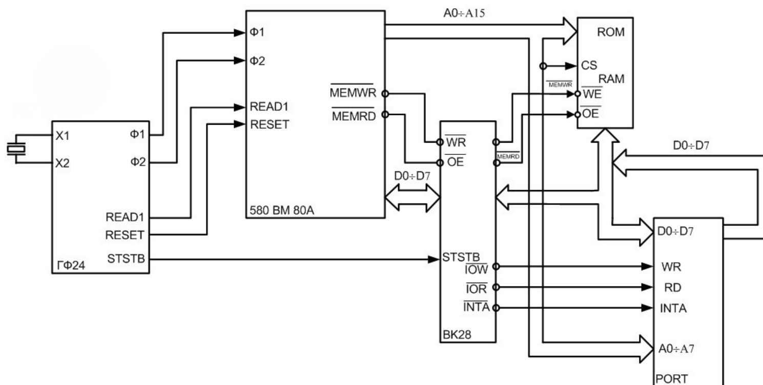
Рисунок 1. Структурная схема микропроцессорного устройства
