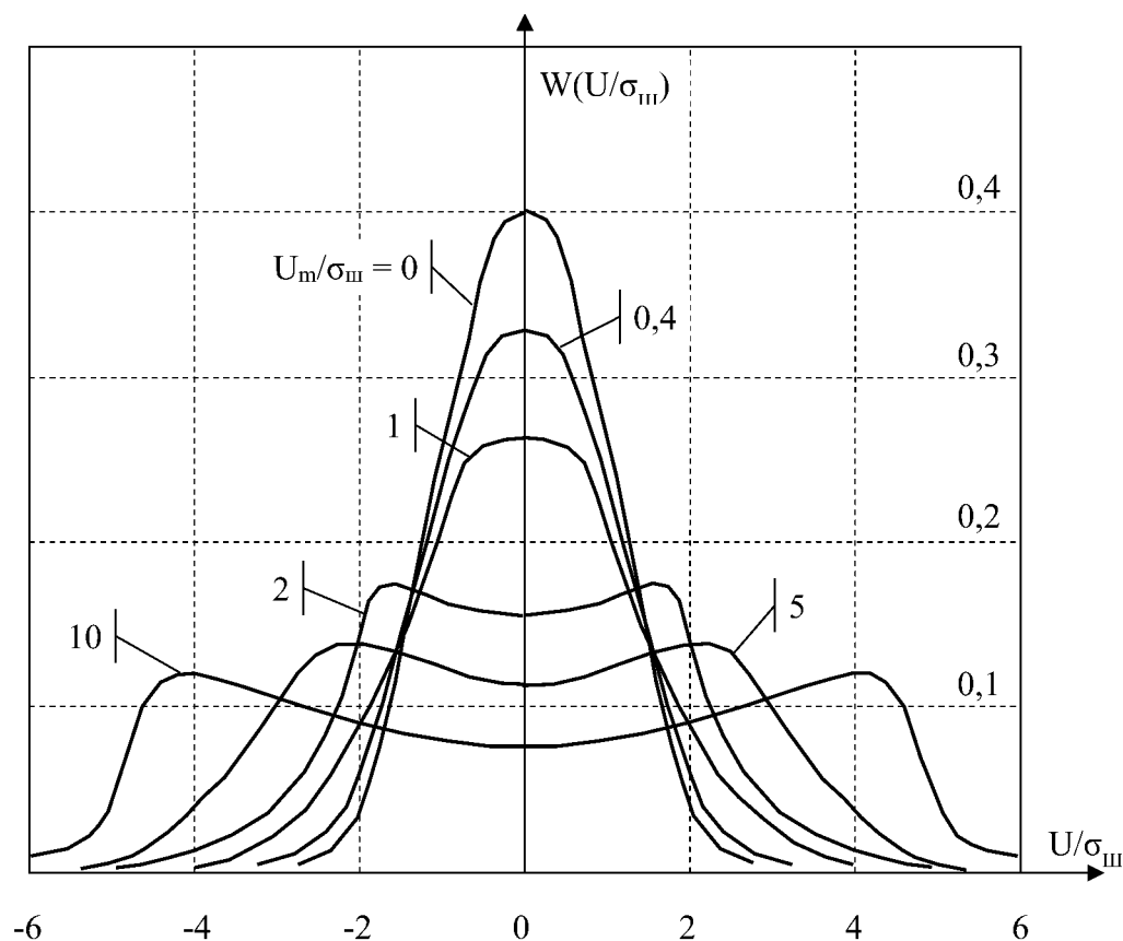
Рис. 8. Функция плотности вероятности смеси сигнала с шумом
