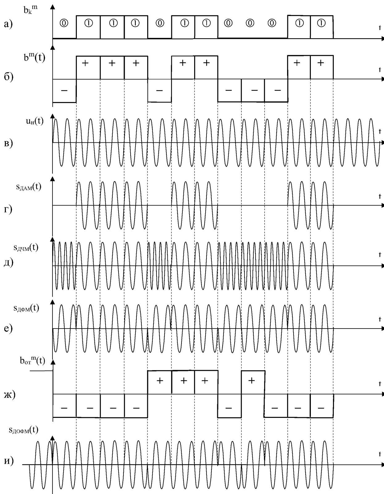
Рис. 7. Сигналы при дискретной модуляции
