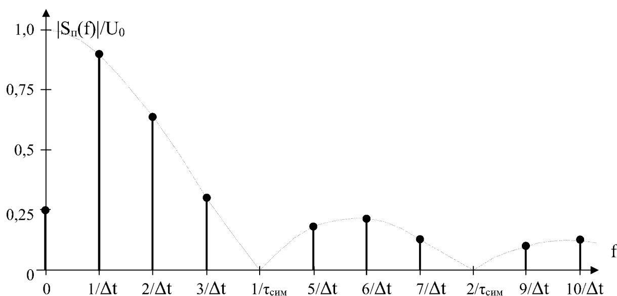
Рис. 6 Амплитудный спектр модулирующего сигнала при \mu = 4
