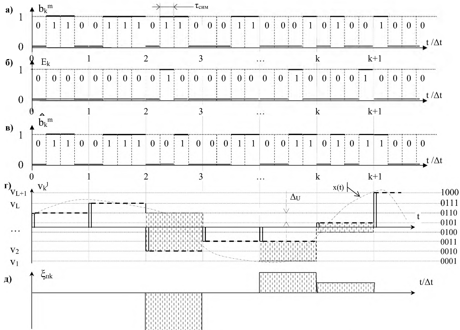
Рис. 10. Восстановление сигнала в ЦАП
