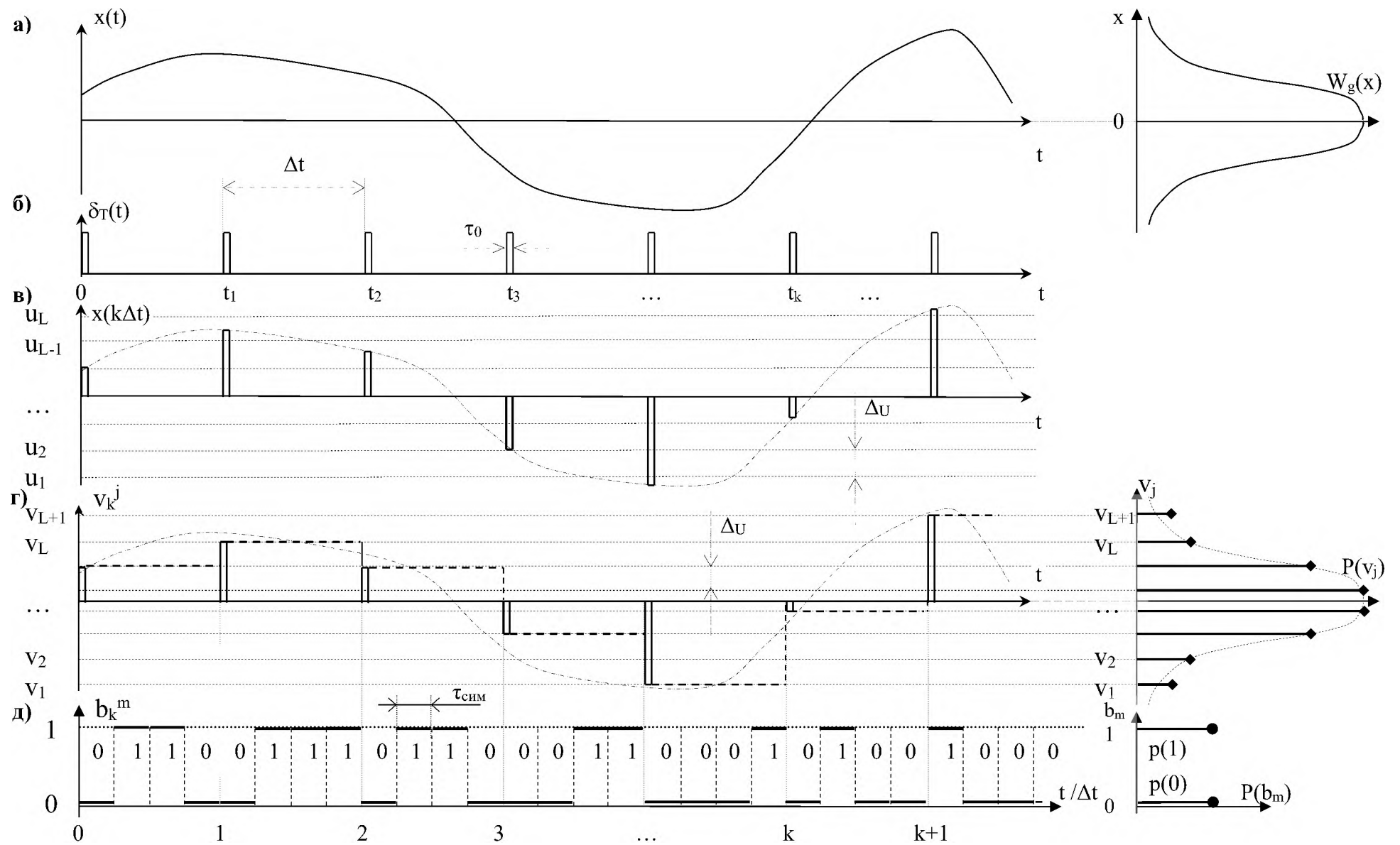
Рисунок 2 Аналого-цифровое преобразование сигнала
