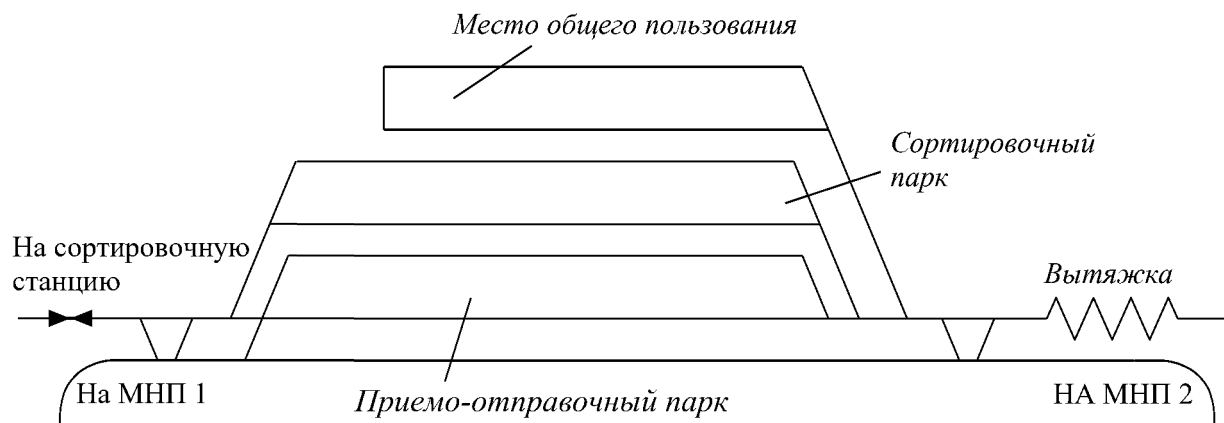
Рис. 1. Схема грузовой станции
