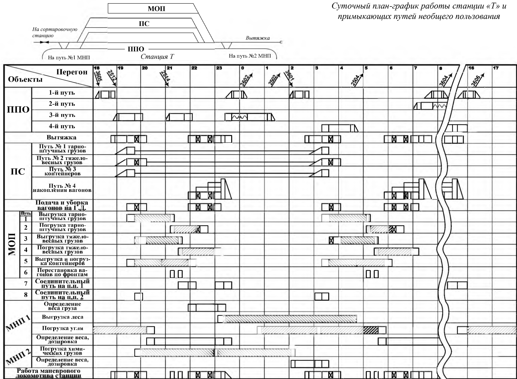
Рис. 2. Суточный план-график
