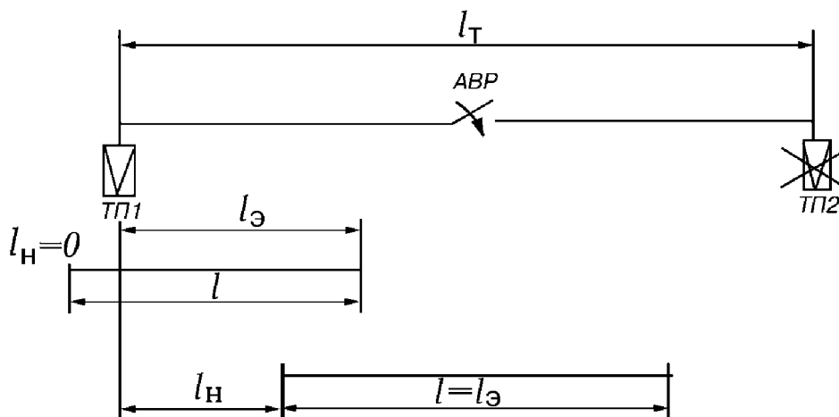
Рисунок 5 – Схема определения длины сближения линии связи с тяговой сетью l_{\text{с}}
