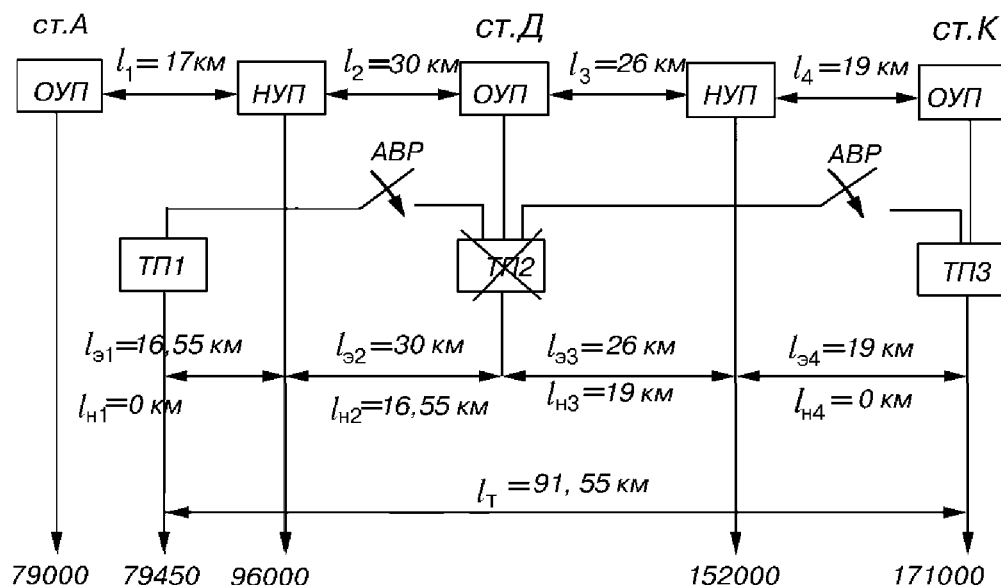
Рисунок 4 – Пример расчетной схемы
