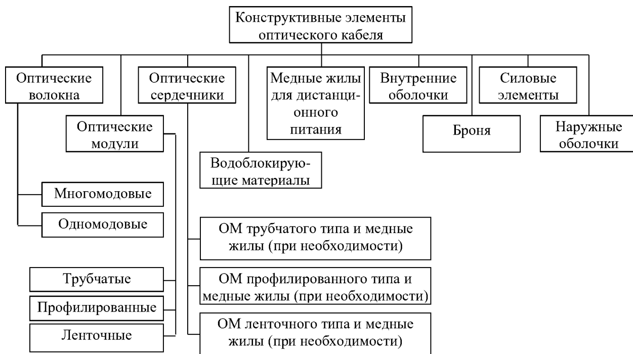
Рис. 7. Основные конструктивные элементы оптического кабеля
