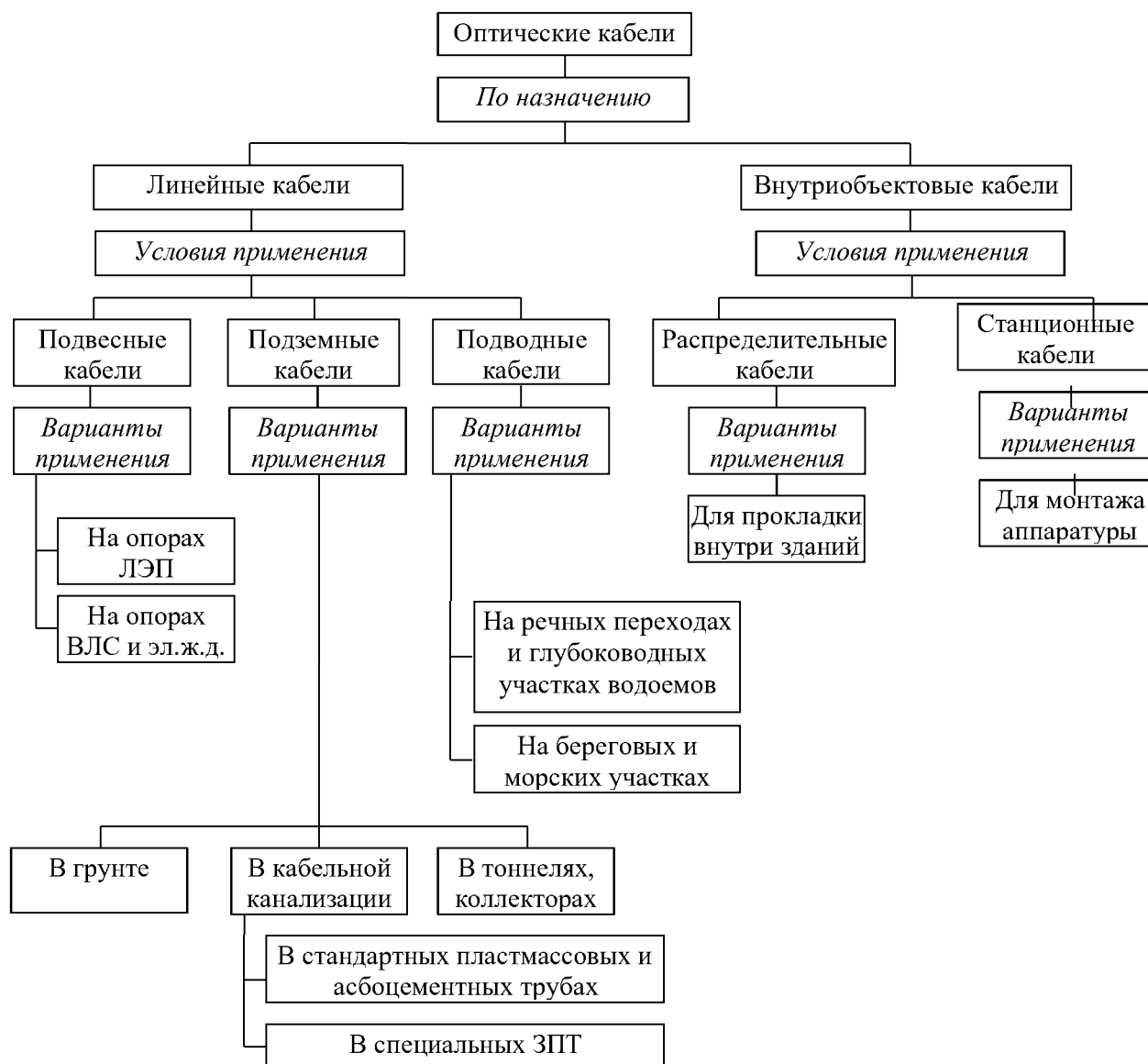
Рис. 6. Классификация оптических кабелей
