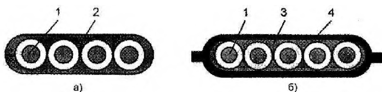
Рис. 9. Примеры конструкций ленточного ОМ: а) с полимерным защитным материалом;
