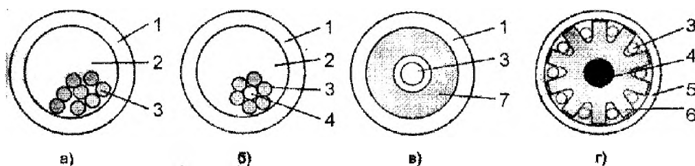
Рис. 8. Примеры конструкций ОМ: а), б) и в) – трубчатых; г) – профилированного.
