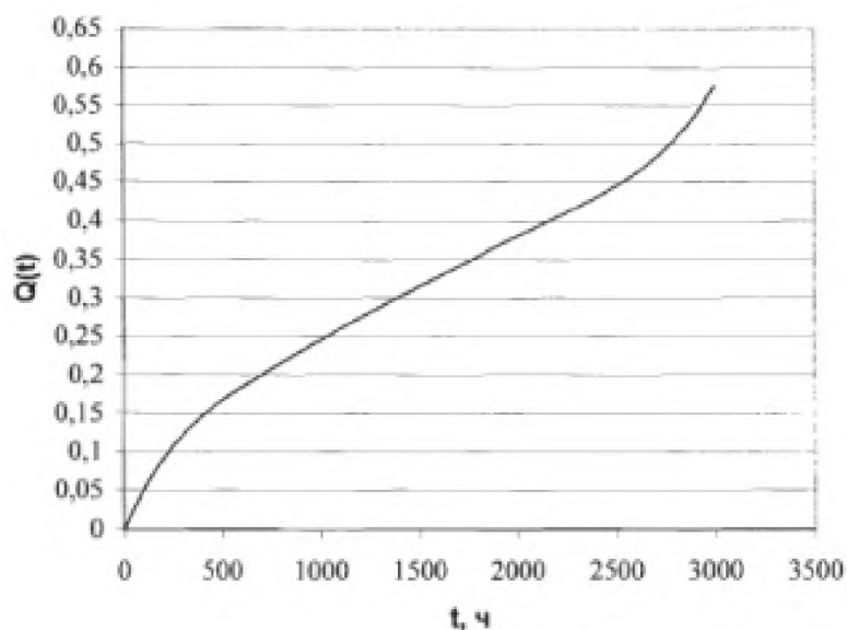
Рис. 1.2. Зависимость вероятности отказов системы от времени Далее определим частоту отказов ситемы на отрезках времени.
