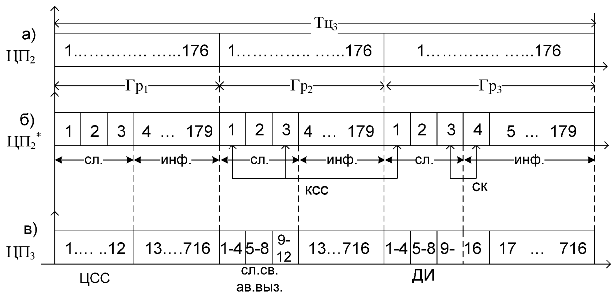
Рисунок 6 – Построение цикла передачи третичного цифрового канала
